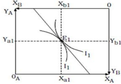
Şekil 2.1: Edgeworth diyagramı
